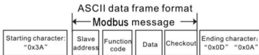
Định dạng khung truyền ASCII
