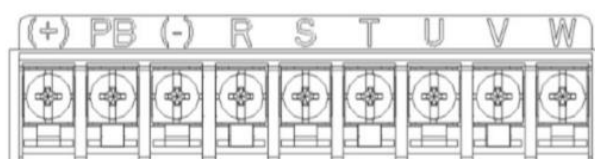
Hình 3-6 3PH Terminal mạch chính (220V, \leq 1.5kW và 380V, 4-22kW)
