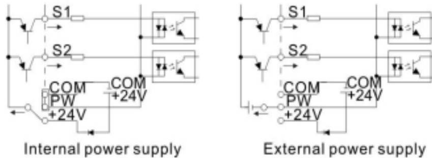
Hình 3-13 Kiểu PNP
